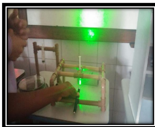
Figura 6.9- Alunos do 2º ano A, mostrando o Microscópio de Gota a laser (A) microscópio com movimento azimutal e (B) modelos diferenciados de PVC.
