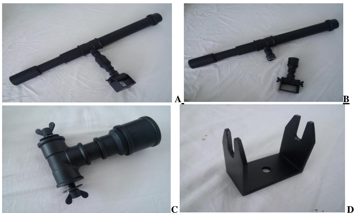
Figura 6.15 – Montagem auto azimutal da Luneta Astronômica (A). Mancal de ajuste para foco horizontal (B). Mancal de ajuste vertical com parafusos borboleta(C). Base de metal em U(D).
