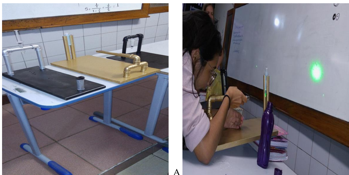
Figura 6.12- (A)Microscópios de gota a laser exposto e (B) aluna manuseando o laser.
