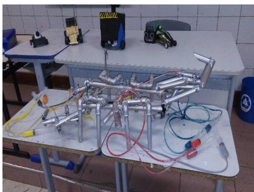
Figuras 6.4 – Guindaste hidráulico (A) Escorpião e (B) Grua.
