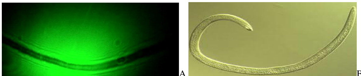
Figura 6.10 – (A) Imagem produzida pelo Microscópio de Gota a Laser de um Nematódeo (imagem própria, 2016) e (B) sua imagem em microscopia óptica.
